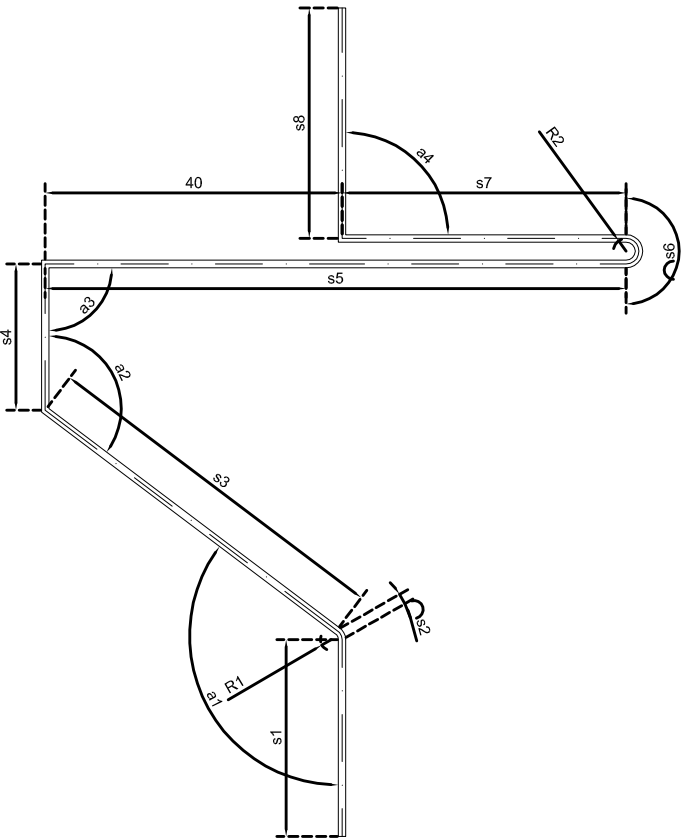
SEZIONE PROFILO "BASE" PROFILE SECTION
