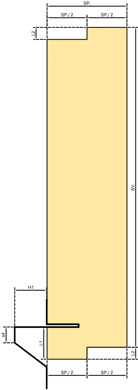
SEZIONE PANNELLO PANEL SECTION
