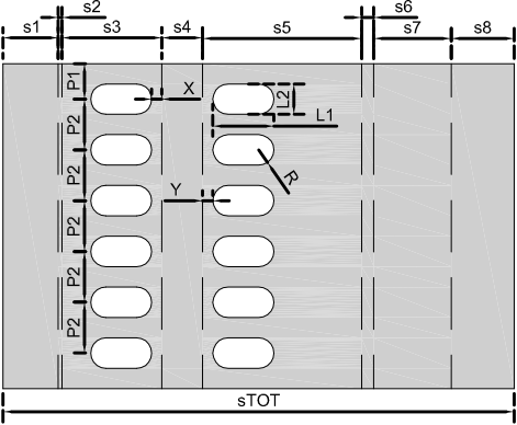
PROFILO "MONTANTE 1" PROFILE
