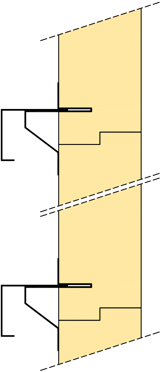
SEZIONE VERTICALE SEQUENZA PANNELLI SECTION
