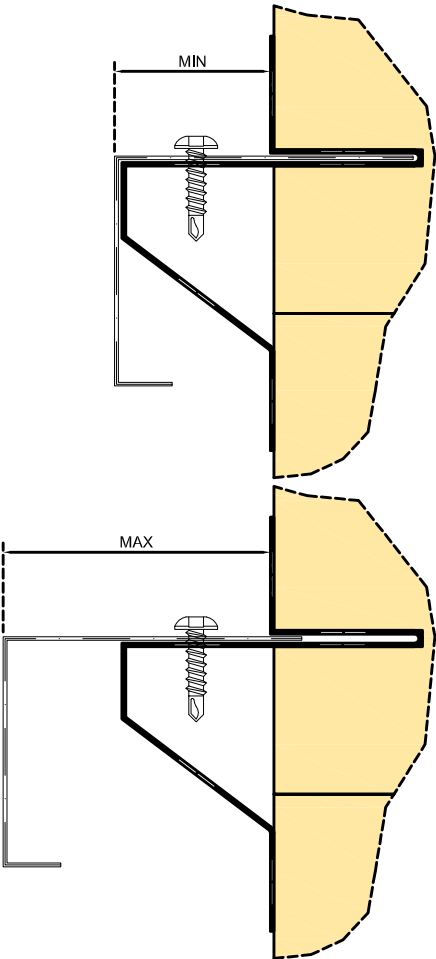
SEZIONI DI MINIMA E MASSIMA ESCURSIONE DEL MONTANTE SECTION
