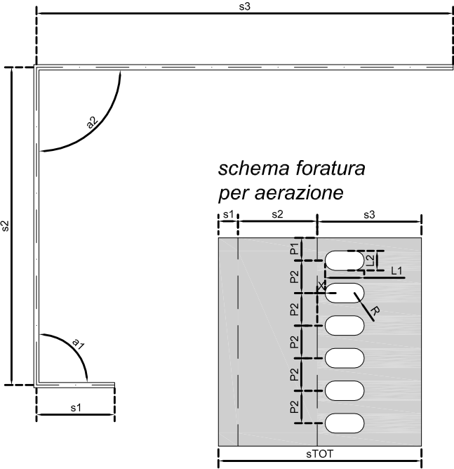
SEZIONI DI MINIMA E MASSIMA ESCURSIONE DEL MONTANTE SECTION
